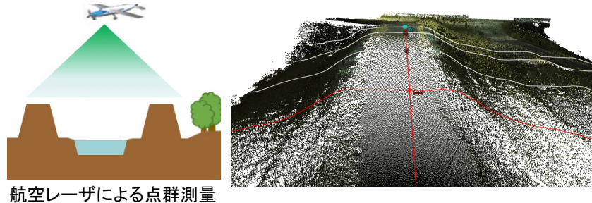
河川縦横断測量（河道の状況把握）
