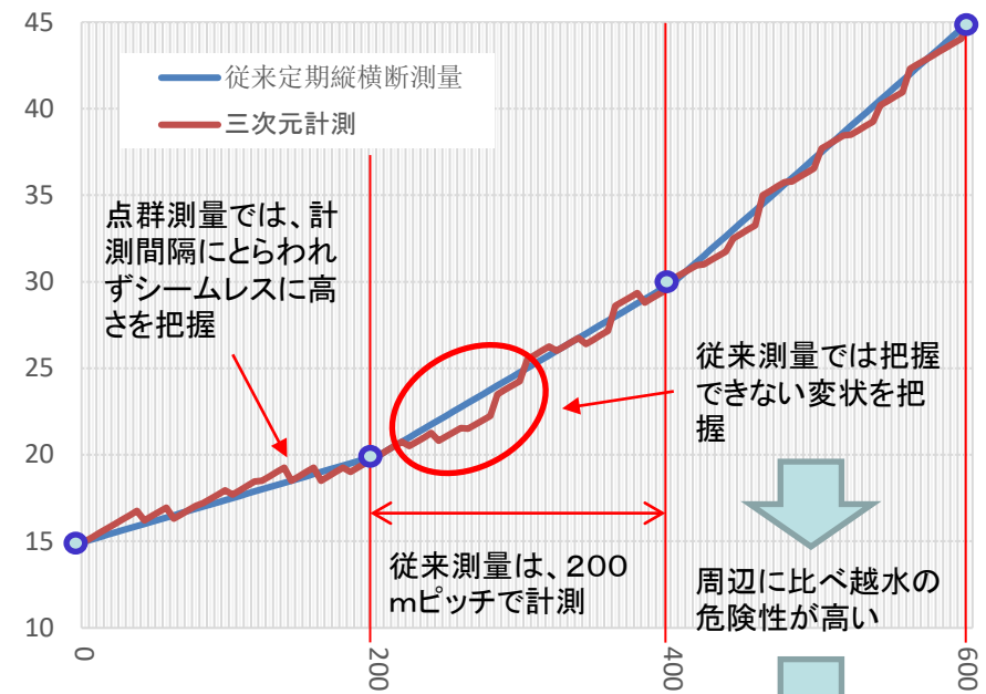
従来測量と点群測量の堤防天端高計測イメージ
