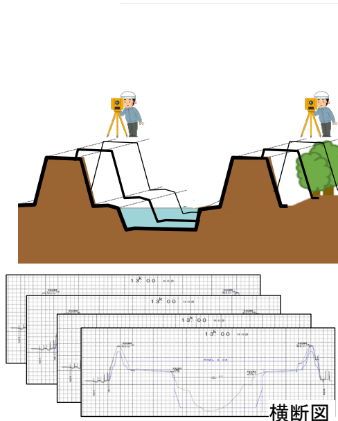
従来の定期縦横断測量
