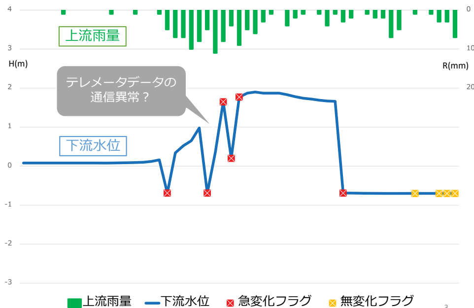
10分水位データチェック <異常検知例-2>
