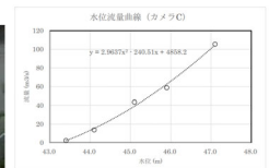
図-5 カメラC地点 (上与市橋上) での水位流量関係
