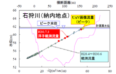
計画高水流量に匹敵する流量の計測に成功
