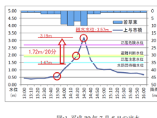
図-1 平成30年7月6日の出水
